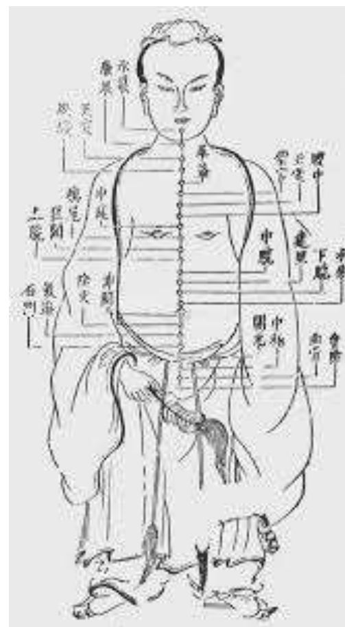
Figura 2. Representação de um merídiano (Frigado, 2003, p.200)
